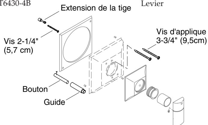
Pièces du kit de raccordement en profondeur
