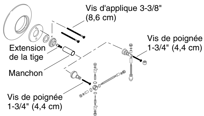
Pièces du kit de raccordement en profondeur
