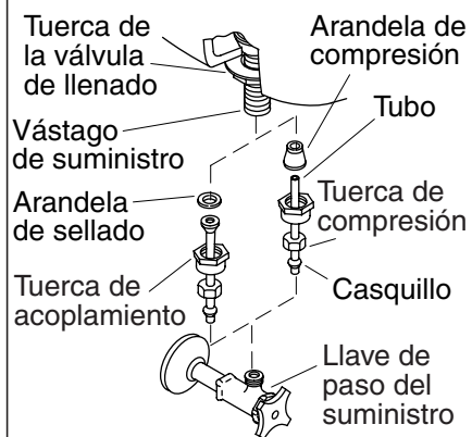
Conexión de la llave de paso del suministro
