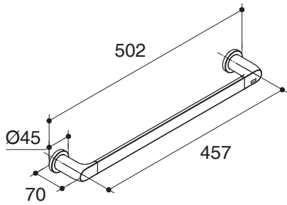
K-97494T
