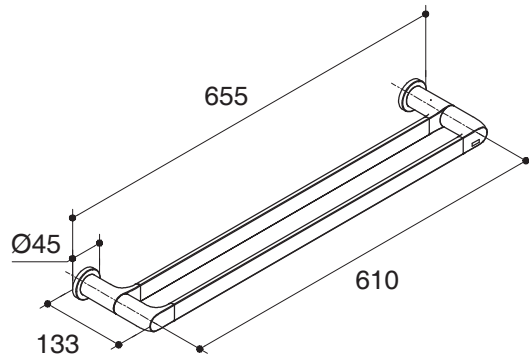
K-97496T
