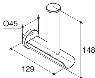
K-97502T
