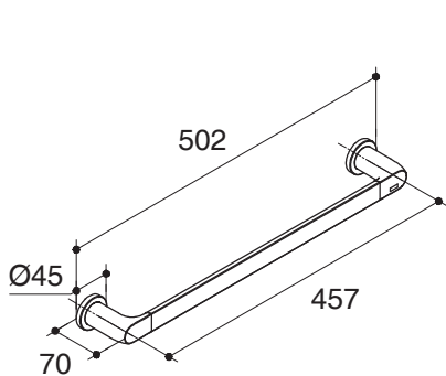
K-97494T
