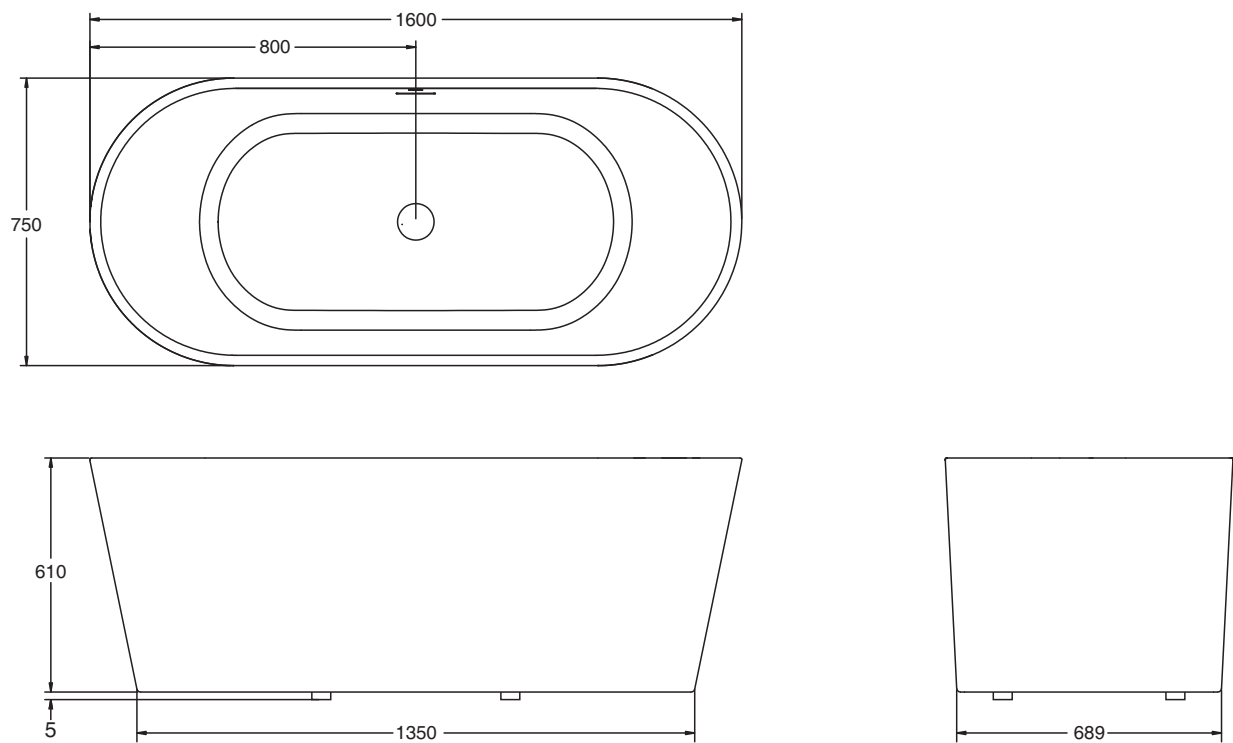
ROUGHING-IN 产品尺寸图 (Unit:mm) (单位: 毫米)
