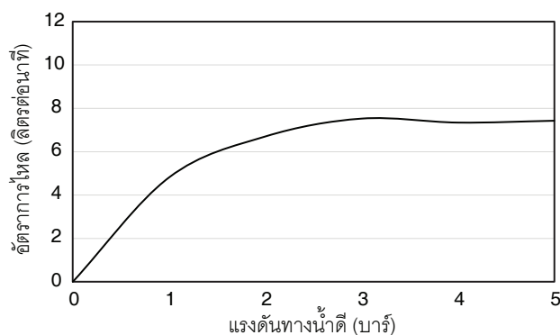
กราฟแสดงอัตราการไหล EX36232T-9WPL / 9BPT
