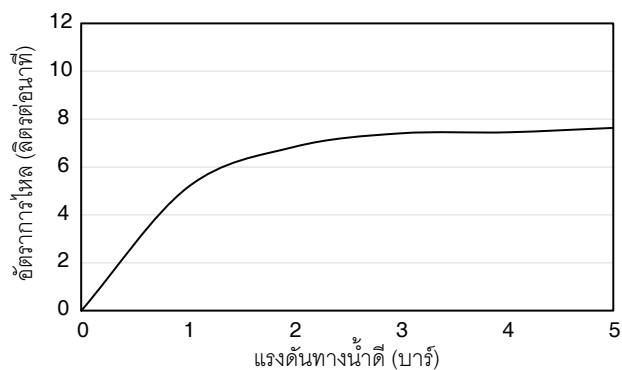
กราฟแสดงอัตราการไหล EX36233T-9WPL / 9BPT
