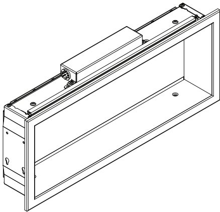
(1) Niche Éclairée CÔV / Nicho Iluminado CÔV
