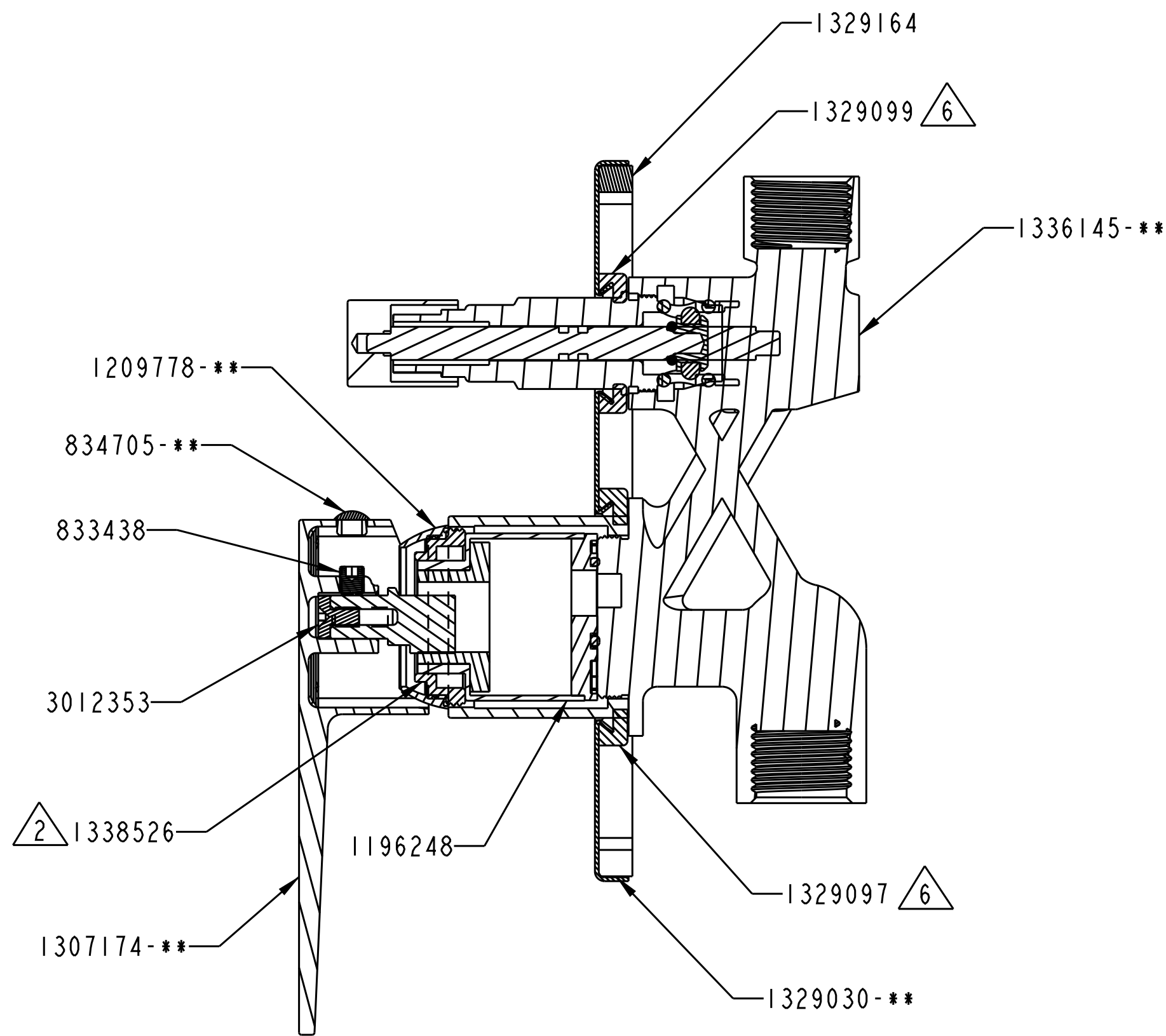
SECTION A-A
