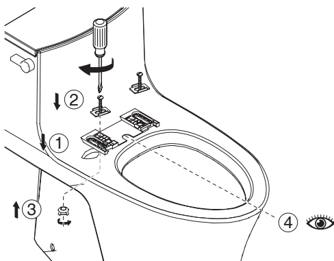
Installation method B / 安装方式 B Hidden Cord / 隐藏管线版
