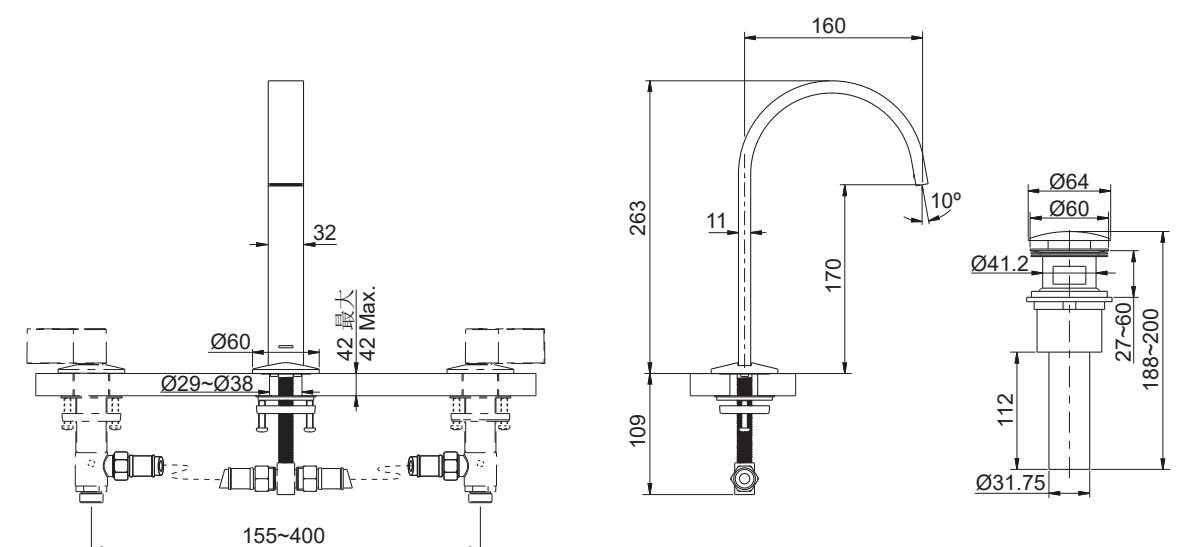
77968T/77968T-MU
