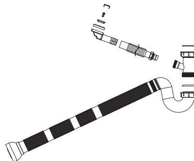
SP1200368-C1 S-Trap 50 (Single basin) ชุดข้อต่อน้ำทิ้ง (หนึ่งหลุม)
