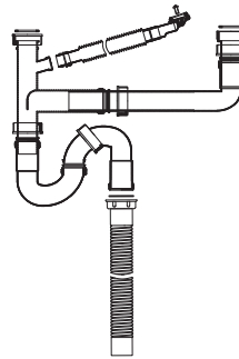
SP1200364 S-Trap (Double Basin) ชุดข้อต่อน้ำทิ้งแบบลงพื้น (สองหลุม)
