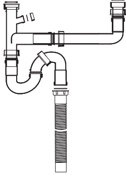
SP1426536 S-Trap (Double Basin) ชุดข้อต่อน้ำทิ้งแบบลงพื้น (สองหลุม)
