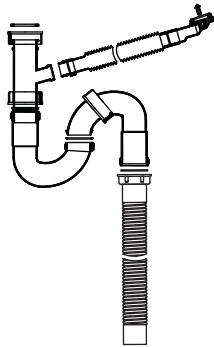
SP1200363 S-Trap (Single Basin) ชุดข้อต่อน้ำทิ้งแบบลงพื้น (หนึ่งหลุม)
